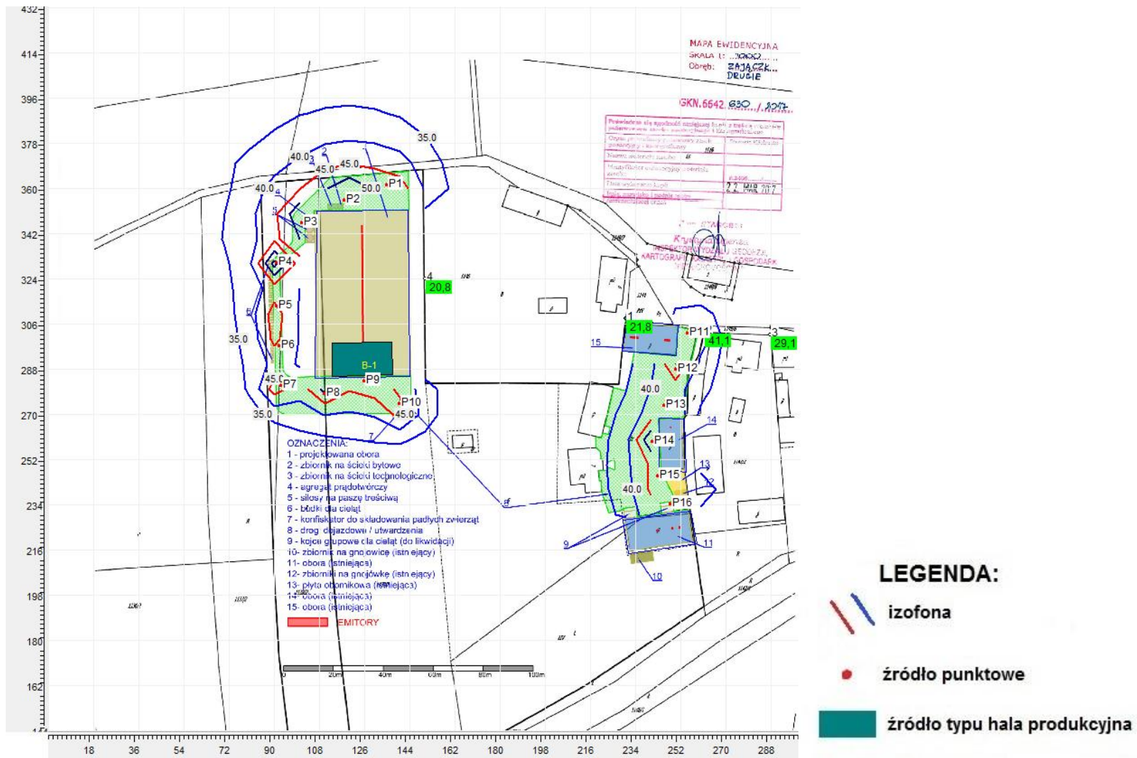
Mapa rozkładu izofon – pora dzienna
